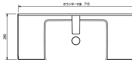
寸法図※2方エプロンの場合
